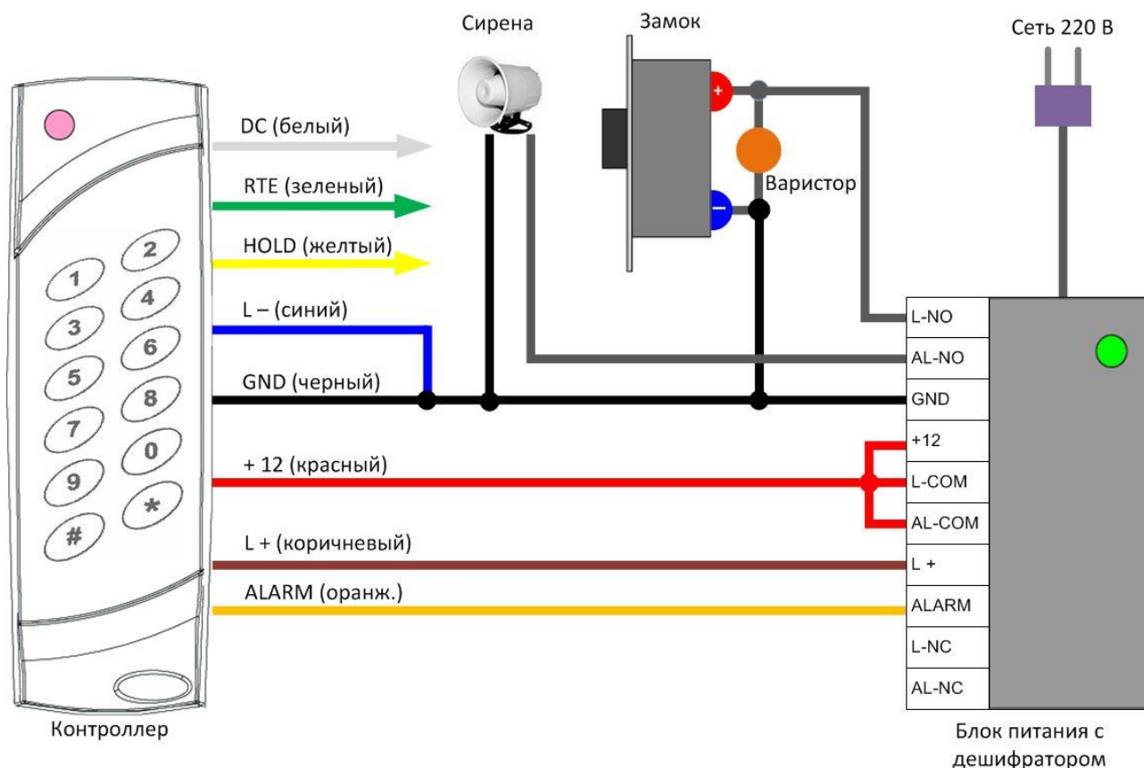
Рисунок 6. Управление замком и сиреной через дешифратор
