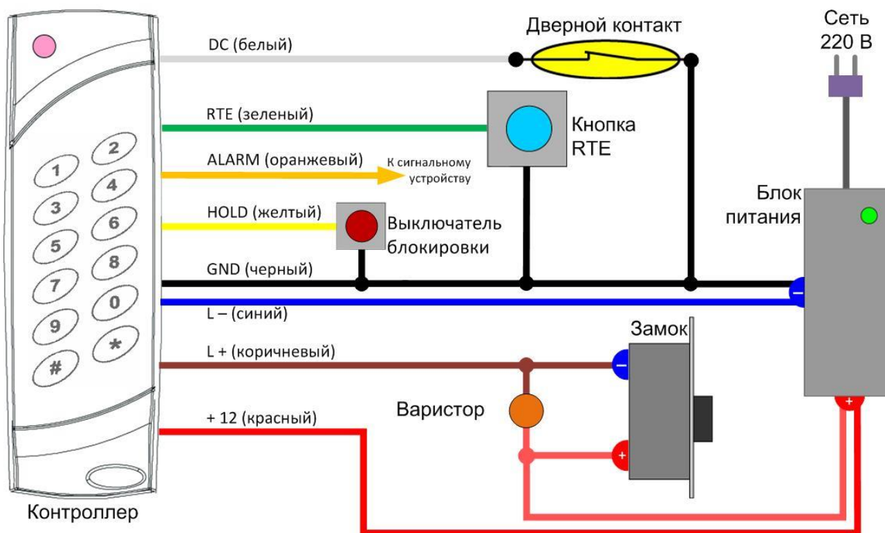
Рисунок 3. Подключение контроллера в заводской конфигурации
