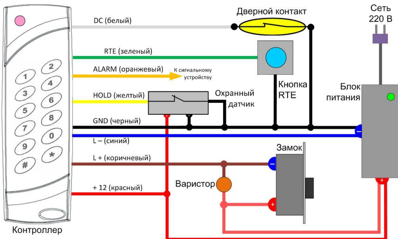
Рисунок 4. Подключение охранного датчика
